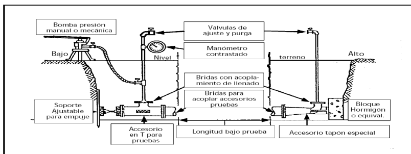
Montaje propuesto para las pruebas de tuberías instaladas
